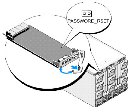
図 12-1. パスワードリセットジャンパの位置
